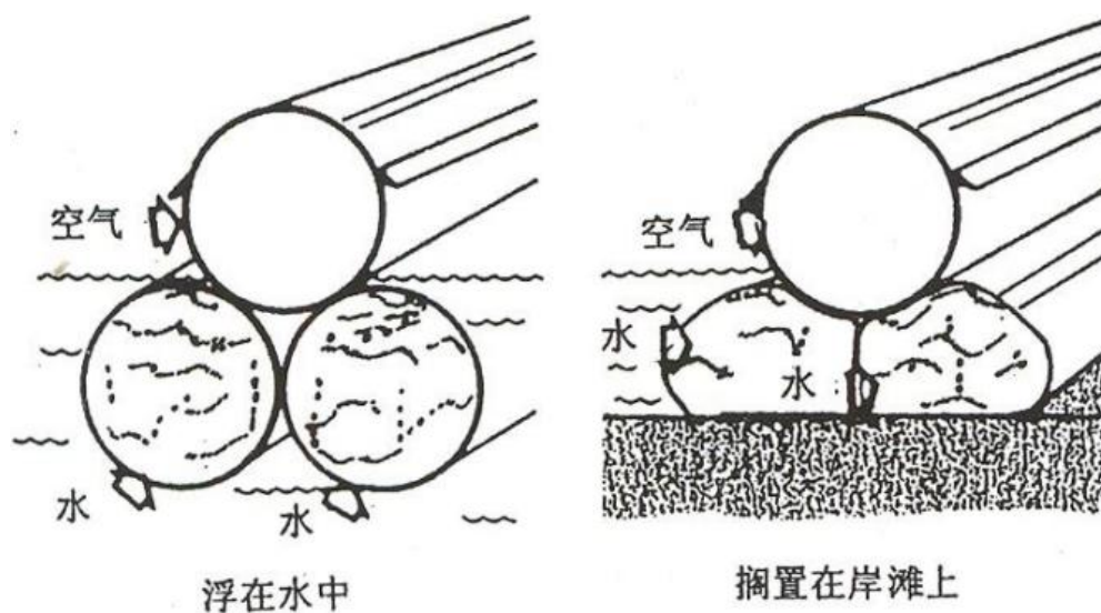
图 4-3 围油栏拦截
